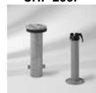
Bodenhülse M4 mit Deckel + Standrohr Stahl verzinkt Stock Ø 48–55 mm CHF 225.--
