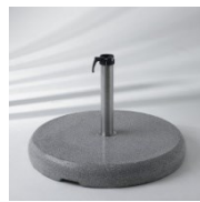
Granitsockel 90 kg Edelstahlrohr Ø 48/55 mm, poliert, Ø 730 mm, poliert, CHF 444.--
