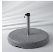
Granitsockel 90 kg Rohr Ø 48/55 mm Ø 730 mm, poliert,
