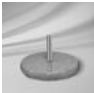
Granitsockel poliert mit Edelst.rohr, 90 kg, Rohr Ø 75 mm
