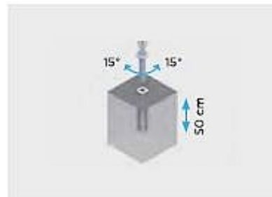
Verstellbare Bodenhülse. Diese Bodenhülse hilft Ihnen mehrere P6 Schirme auf einer gerade Linie zu installieren. Diese Bodenhülse gibt Ihnen einen Freidum von bis zu 15° links und auf den rechten Seite
