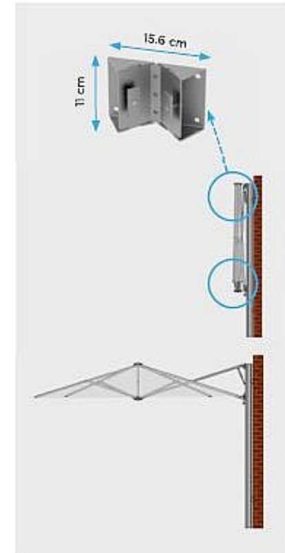
Einfach zu montierende Wandhalterung (2 Stück). Nur möglich für Quadrat P6 Uno oder P6 Duo. Aus unlackiertem, verzinktem Stahl. Weitere Infos auf S. 18
