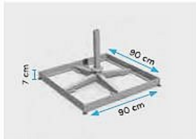
Schirmsockel aus Stahl Mit 8 Fliesen: 130 kg Mit 12 Fliesen: 185 kg Nicht geeignet für XL-Version Ohne Fliesen
