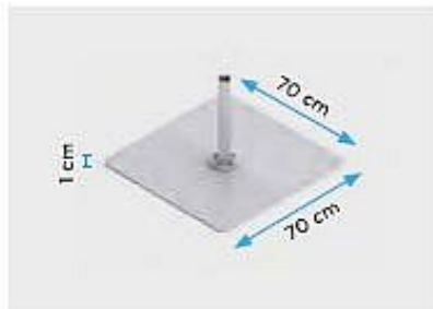
Bodenplatte muss chemisch verankert sein. Gewicht: 38 kg Ohne Befestigungsmaterial geliefert
